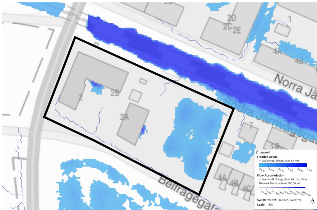
Figur 12 Skyfallsanalys för 100-års regn med klimatfaktor 1,25 och varaktigheten 6h (Nettonederbörden är 64 mm)
