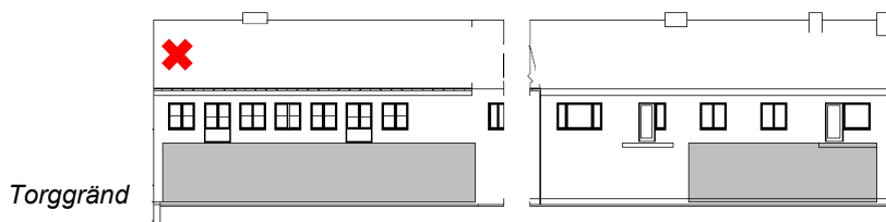
Vy mot norr. Rött kryss markerar vart det inte är tillåtet att uppföra takkupor med hänsyn till bestämmelse f4.
