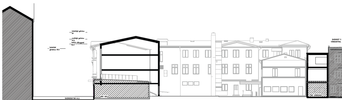
SEKTION B - B
