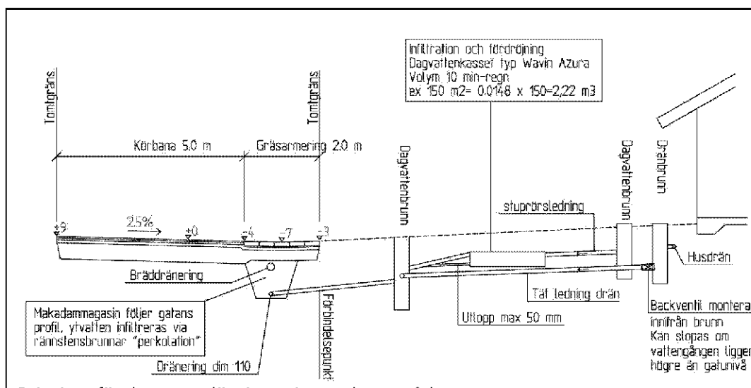
Principer för dagvattenlösningar inom planområdet
