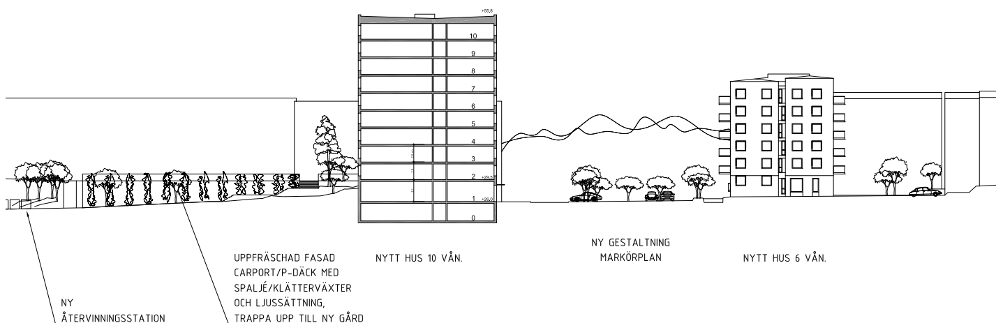
Sektion C-C
