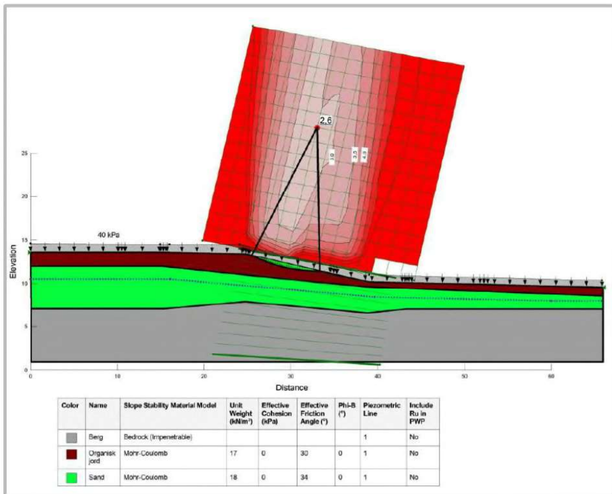
Figur 7: Överslagsmässig stabilitetsberäkning.
