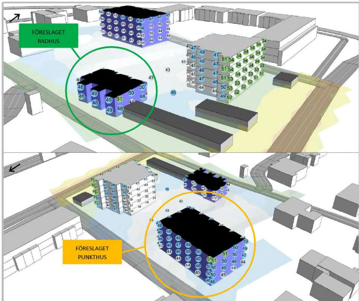
Figur 15: Utdrag ur bullerutredningen, för ekvivalent ljudnivå. Gul ring visar föreslaget punkthus och grön ring föreslaget radhus.
