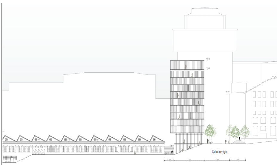
Elevation mot sydväst som visar möjlig utformning och gestaltning av en ny byggnad inom delområde 4. Bild: Kjellander & Sjöberg
