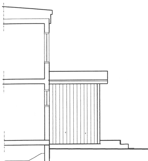
SEKTION/FASAD
