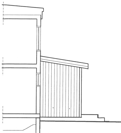
SEKTION/FASAD
