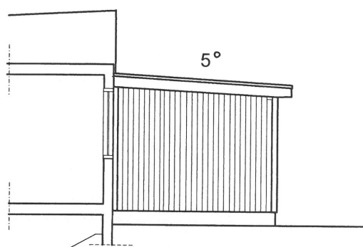
SEKTION / FASAD
