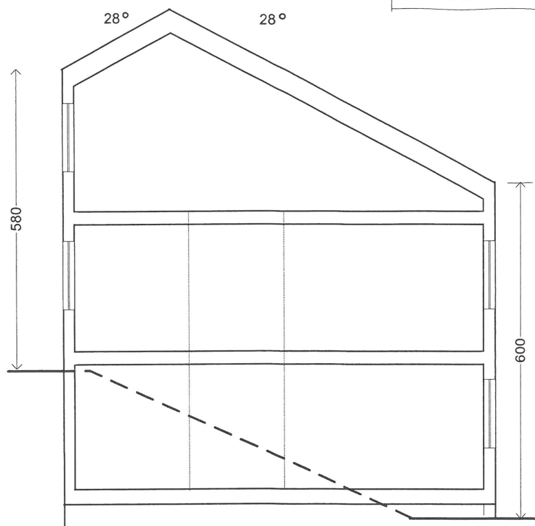
PÅBYGD VÅNINGSPÄN SKALA 1:200
