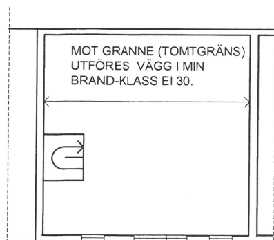
PÅBYGD VÅNINGSPÅN SKALA 1:200
