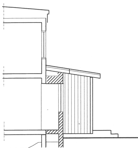
SEKTION / FASAD
