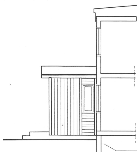
SEKTION/FASAD
