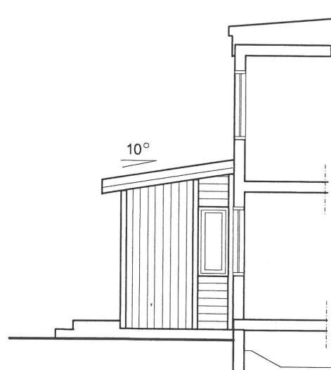
SEKTION/FASAD
