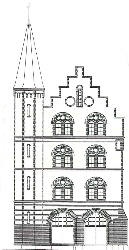
FASAD MOT BORGMASTARGATAN
