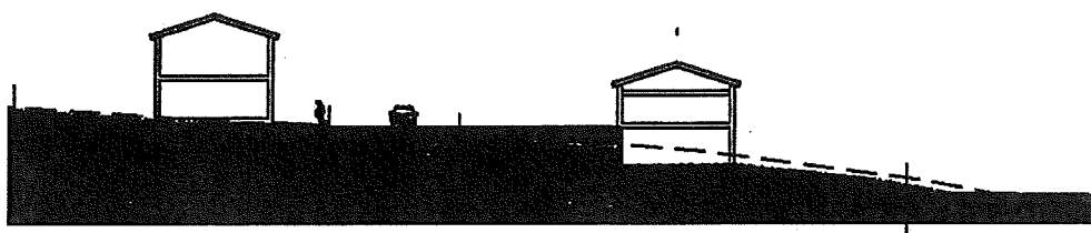
Principsektion B-C genom tomterna längs med gatan i öster
