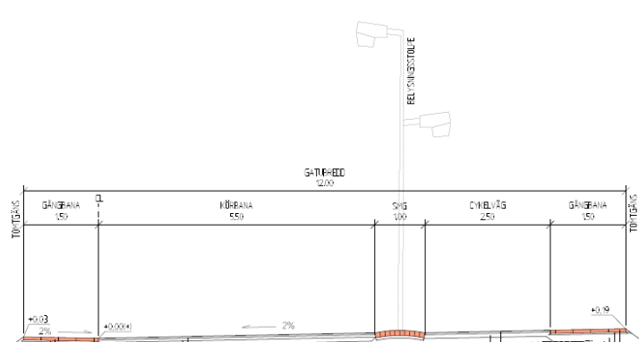
Föreslagen sektion över Framtidsstigen. Föreslagen sektion Planetgatan.
