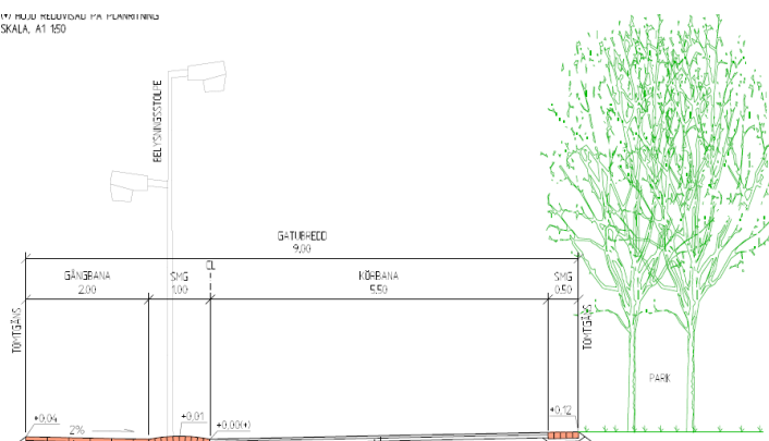
Föreslagen sektion över Insidesgatan.
