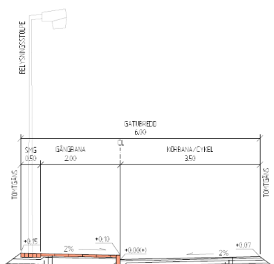
Föreslagen sektion över Framtidsstigen. Föreslagen sektion Planetgatan.
