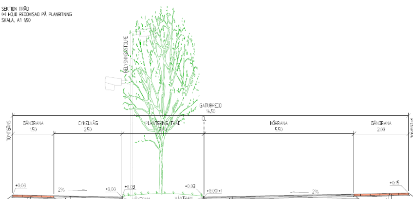
Föreslagen sektion över Regnbågsgatan.
