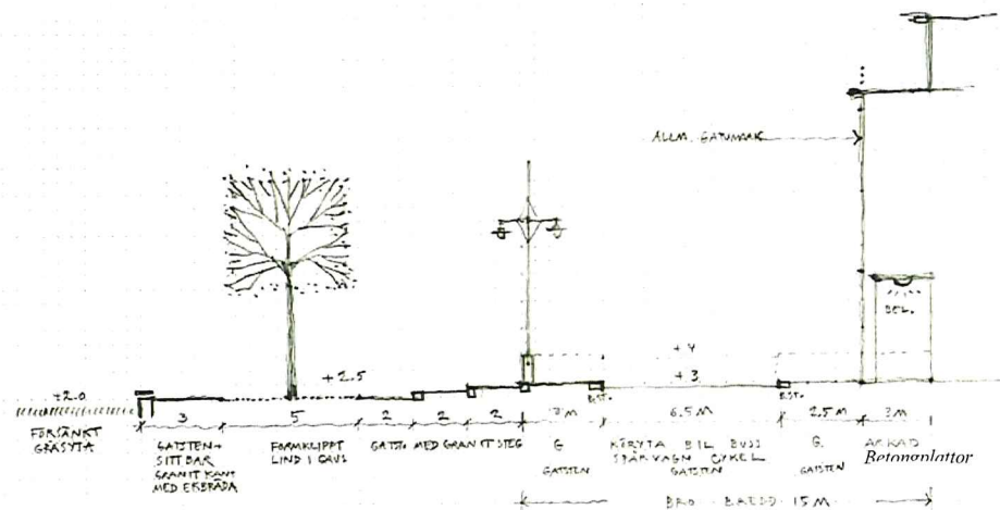
(G1) SEKTION GENOM BRO RAMP VID HAMNTORGET 1:100 27.3.2002 B&FARK/Henrik Farkas REV 9.1.8003
