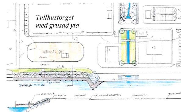
Sektion genom brygga och torg
