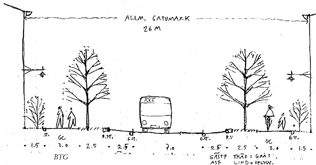
Typsektion, Hamnalléns södra del
