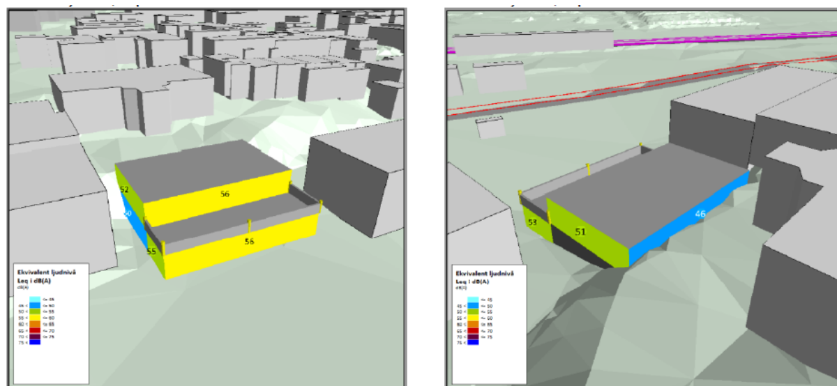
Bild 13: Beräknad ekvivalent bullernivå vid fasad år 2040 (efterklang 2023)
