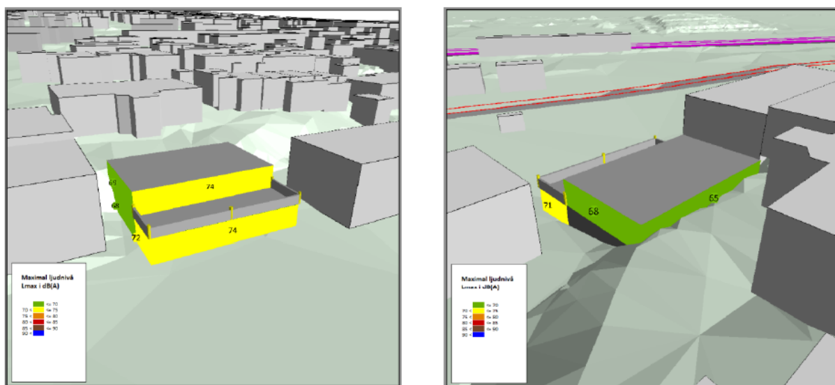
Bild 15: Beräkningar av maximal bullernivå vid fasad för år 2040 (efterklang 2023)
