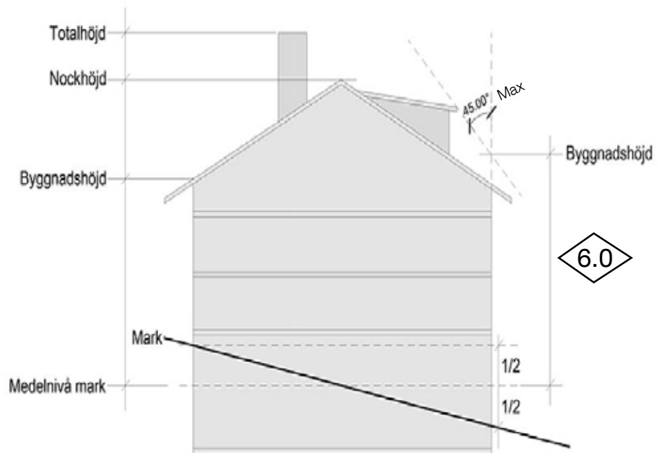
Bilden illustrerar vad som är byggnadshöjd på en byggnad.
