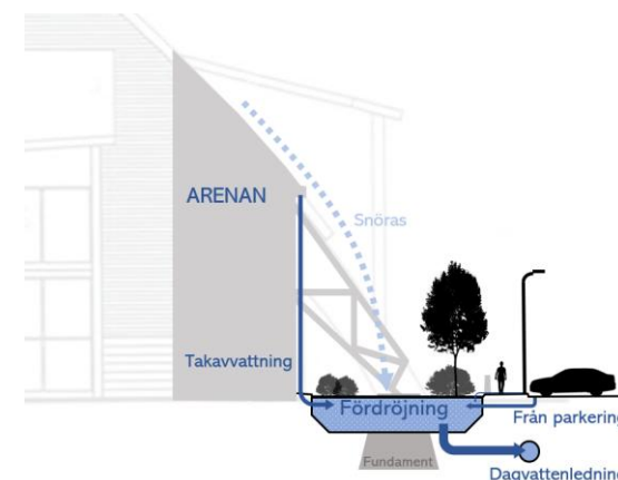
Principskiss på fördröjning av takavvattning och dagvatten från parkeringen vid arenan.
