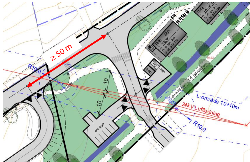
Figur 10. Plats för en ny lokalgata mot området söder om gamla banvallen. Illustration visar möjlig användning av ytor. (2023)
