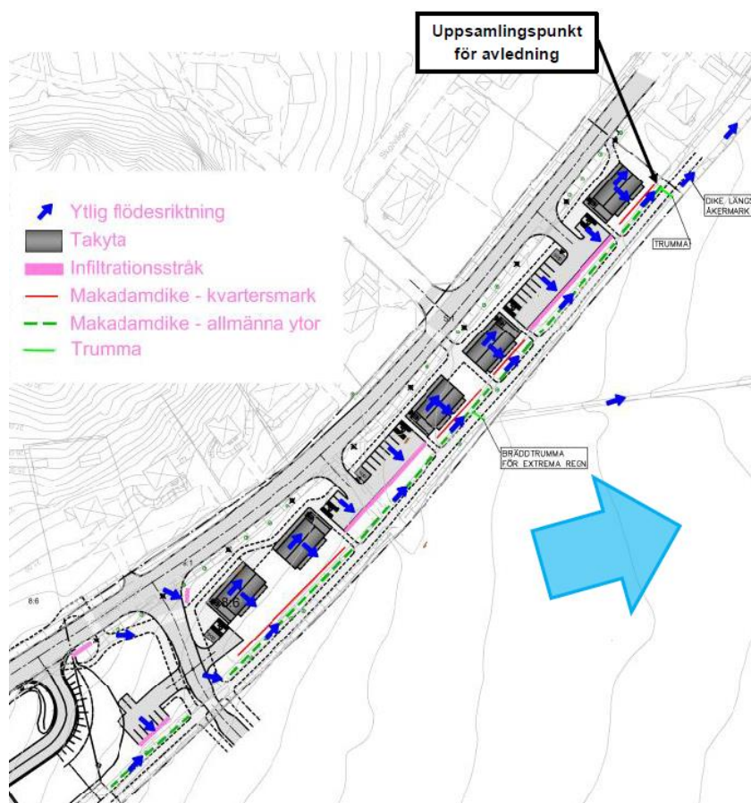
Figur 14. Föreslagen placering av dagvattenåtgärder samt ytor och ytlig flödesriktning (källa: Dagvattenutredningen, WSP Sverige AB, rev. 2024)
