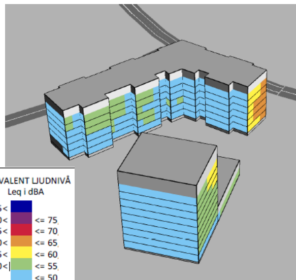
Ljudutbredning innergård fasad år 2040. Ekvivalent ljudnivå.
