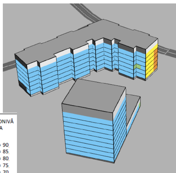
Ljudutbredning innergård fasad år 2040. Maximal ljudnivå.
