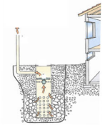
Exempel på luftnings- och tillsynsbrunn för gas.
