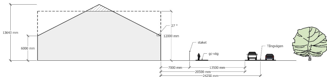
Gatusektion Tångvägen
