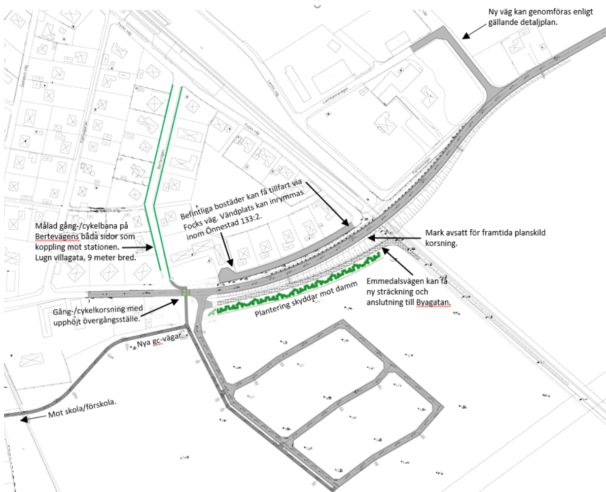
Vägprojektering och redovisning av ytor för framtida planskild korsning. Kristianstads kommun dec 2019.
