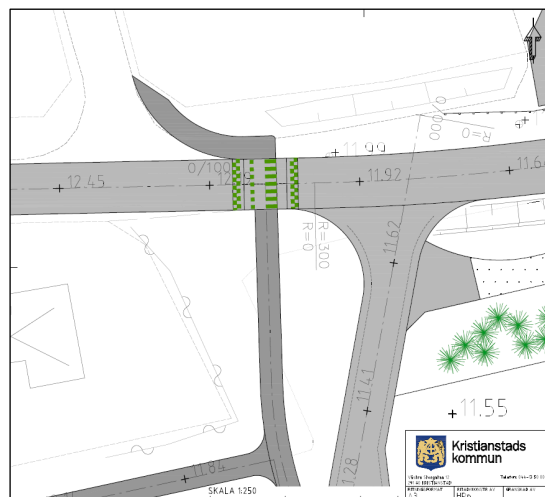
Projekteringsunderlag som visar vägenslutning mot Byagatan samt ny gång- och cykelväg och upphöjt övergångsställe. Kristianstads kommun dec 2019.
