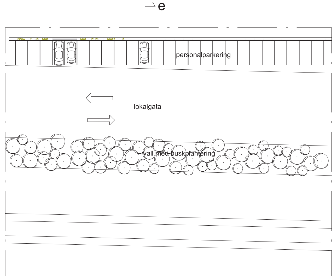
del av plan, obs! annan skala
