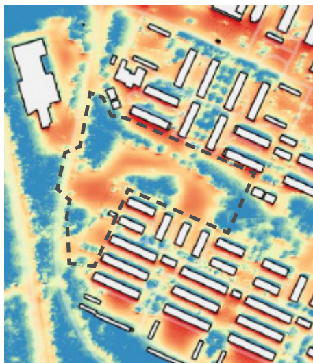
Scenario för ett 2 grader varmare klimat baserat på juni-augusti 2014. Strålningstemperaturen presenteras som antal timmar x antal grader > 55 grader C. (Raport nr 2018-4 Värmekartläggning, Skövde tätort)
