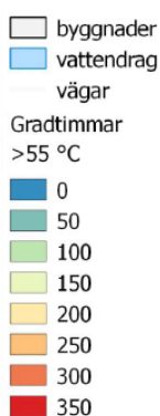
Scenario för ett 2 grader varmare klimat baserat på juni-augusti 2014. Strålningstemperaturen presenteras som antal timmar x antal grader > 55 grader C. (Raport nr 2018-4 Värmekartläggning, Skövde tätort)
