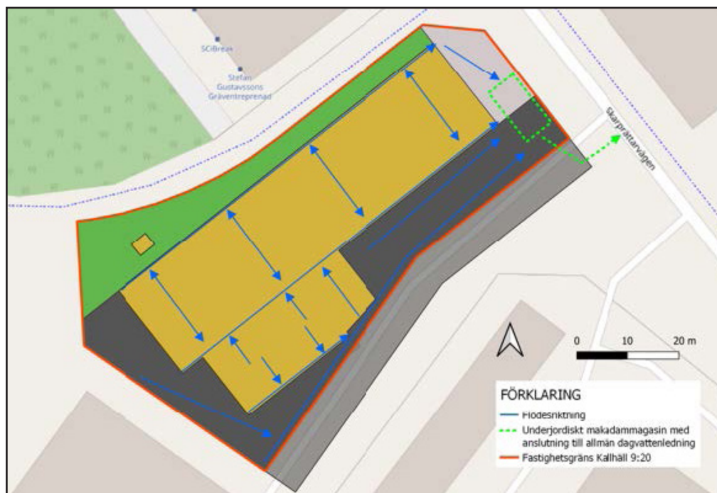
Bild över föreslaget dagvattensystem där hela fastighetens avrinning leds till ett underjordiskt makadammagasin. (Geoveta, 2021).
