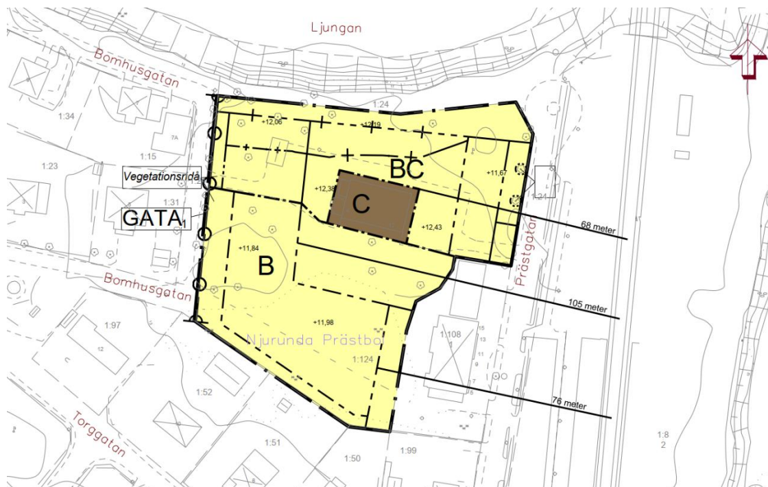
Figur 13. Avstånd mellan järnvägen (spår) i öster och befintlig byggnad (Prästgården) samt förslag på tillkommande byggrätt i den södra delen av planområdet.
