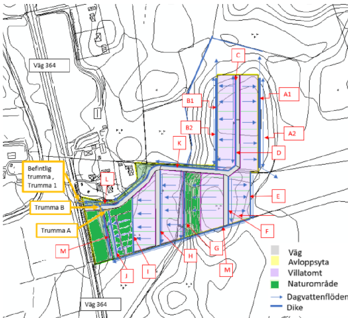
Figur 25. Ugefärlig skiss över dagvattenflöden och rinnvägar
