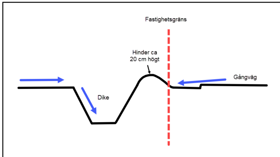
Illustration ur dagvattenutredning. Principskiss på en tvärsektion av diket och gångvägen. Skissen är inte skalenlig.
