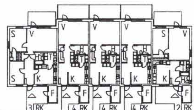
ENTRÉPLAN
