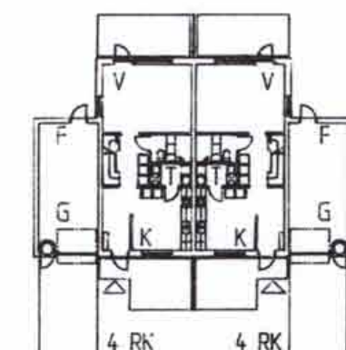
ENTRÉPLAN
