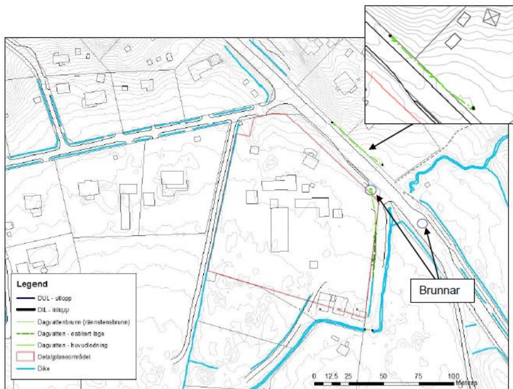
Figur 4. Befintliga dagvattenledningar och diken i anslutning till planområdet samt två dagvattenbrunnar som noterades vid platsbesök (Atkins 2015).
