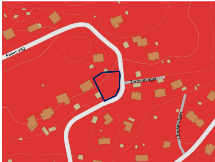
Bild från SGU:s hemsida som visar de översiktliga geotekniska förhållandena inom berörd fastighet. Röd färg visar urberg. Planområdet är markerat med blå linje.
