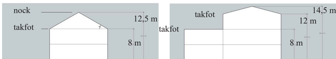
Bild 16: Principskiss på hur byggnadernas höjder regleras. Förskjutning i nock och varierade takfotshöjder får medges. Viss förskjutning i fasad får också medges med högre fasadhöjd som konsekvens förutsatt att detta inte dominerar byggnadens uttryck och påverkar byggnadens skala negativt.
