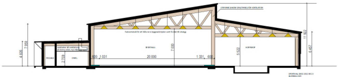
Bild 15: Sektion av skolans idrottshall med gymnastikdel, förråd och omklädningsrum. Liljewalls arkitekter 2022-09-07.
