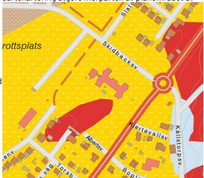
SGU:s jordartskartering, glacial finlera (gult) och berg (rött)
