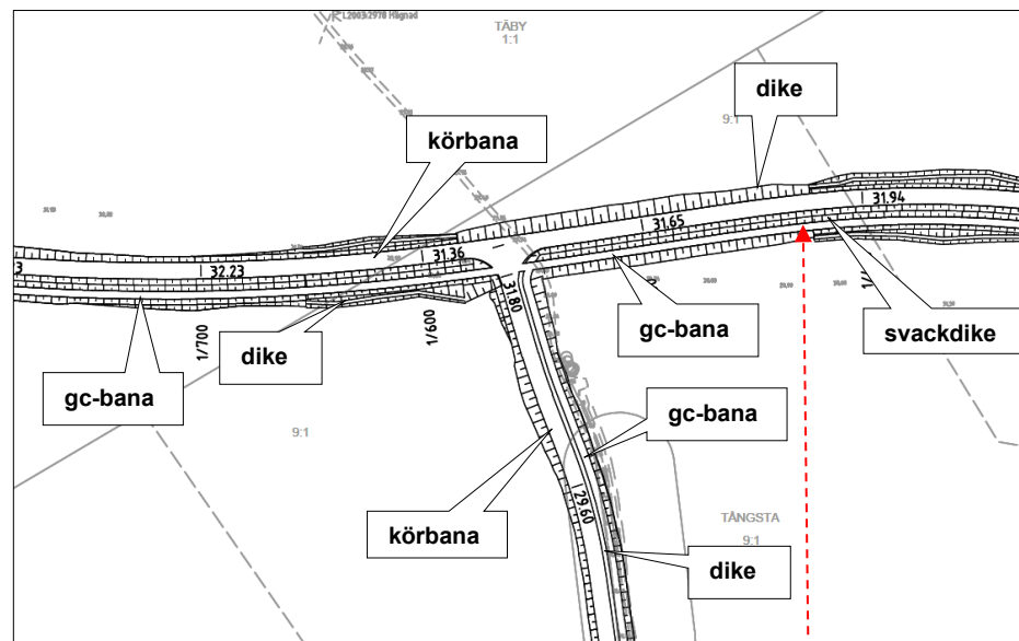
Figur 8. Vägområde. Utsnitt ur vägförprojektering, förlängning av Gäddeholmsvägen (Väg och VA ingenjörerna, 2023)
