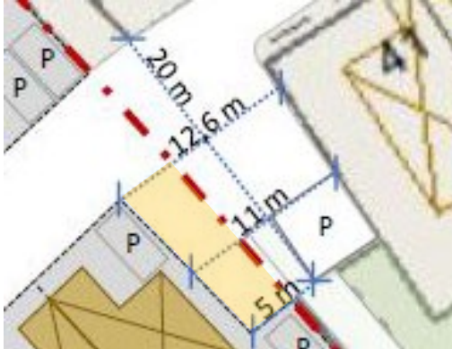
Illustration: Dimensionering av utökad vändzon. Gulmarkerad yta visar ytan som läggs till den befintliga vändzonen. Angivna mått är avrundade till närmaste tiondels meter.
