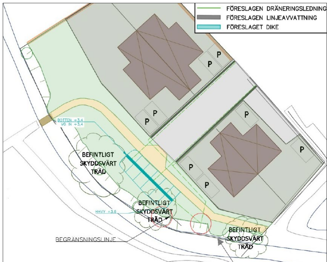
Illustration: Förslag på schematisk utformning av dike vid dagvattensystem i form av linjeavvattning och separat dräneringssystem (Ramboll, 2025).
