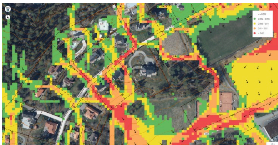
Utsnitt ur Sigtuna kommuns skyfallskartering. Beräknade maximala vattendjup (m) för ett 100 års regn med klimatfaktor 1,25
