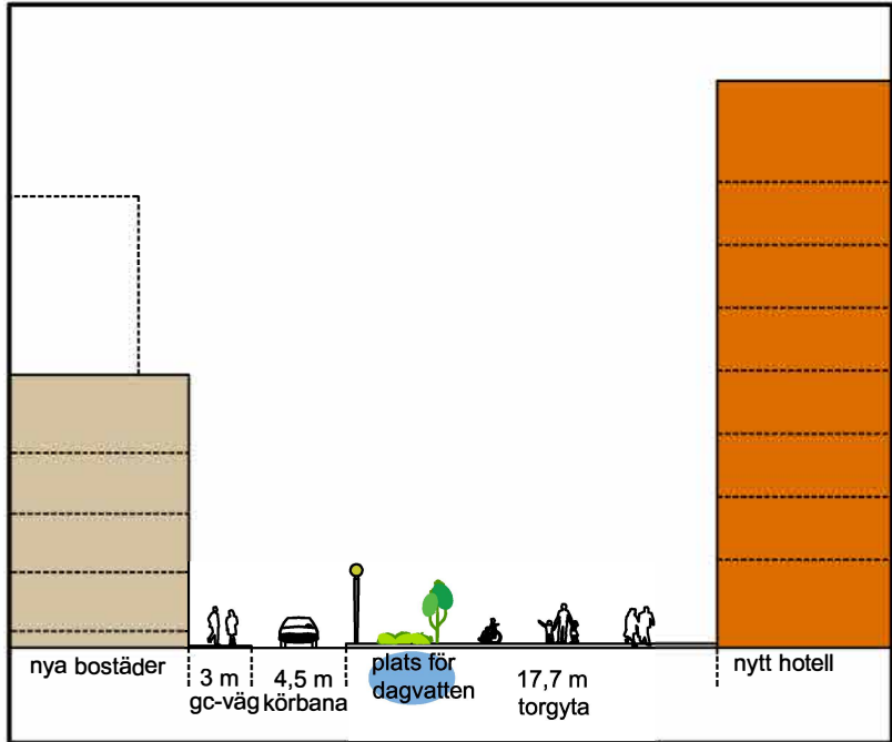
En sektion över hur torget kan utformas.
