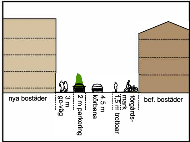
En sektion över hur Helmfeldtsgratan kan utformas
