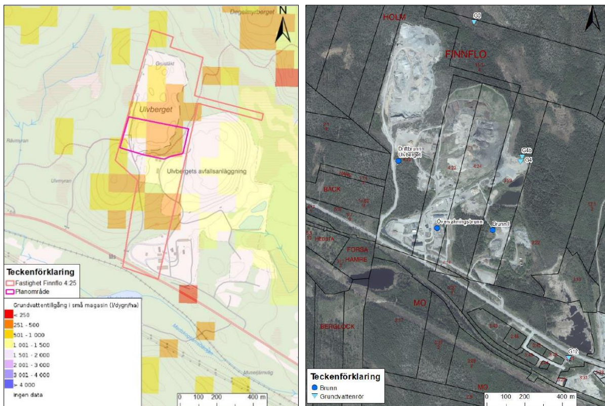
Figur 12, Grundvattentillgång (till vänster) och hydraulisk konduktivitet (till höger). Figur 13, Befintliga brunnar och vattenrör i området kring Finnflo 4:25.
