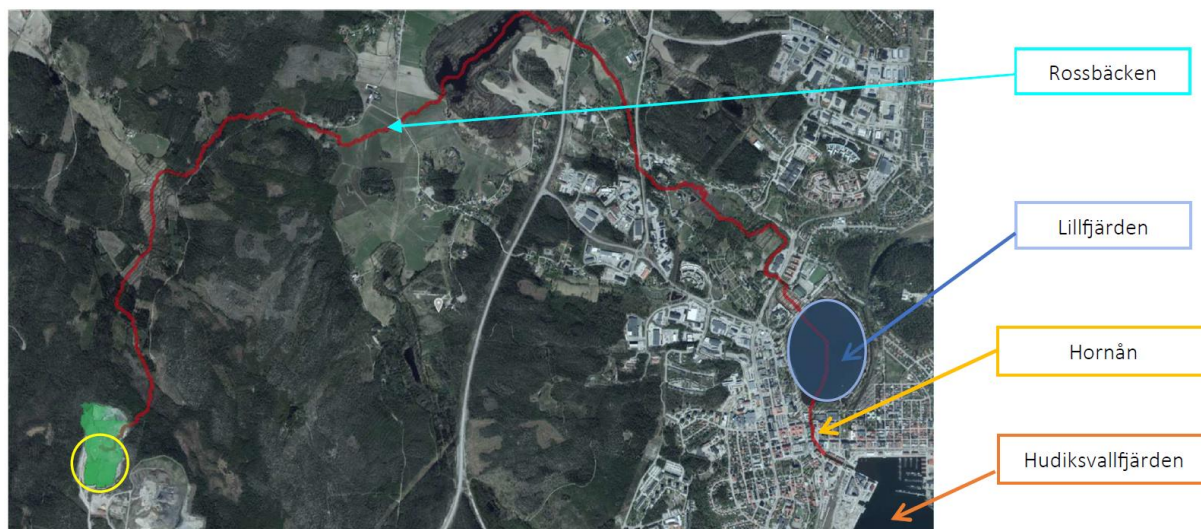
Figur 10, Översiktsbild från Scalgo med avrinningsområde markerat i grönt, planområde markerat med gul cirkel och ytavrinningsväg i rött.
