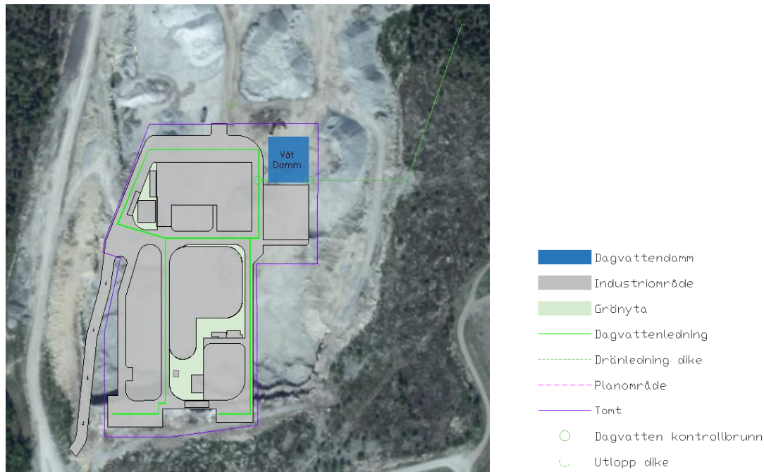
Figur 2, översiktlig illustration över verksamheten med föreslagna dagvatten- och dräneringslösningar.
