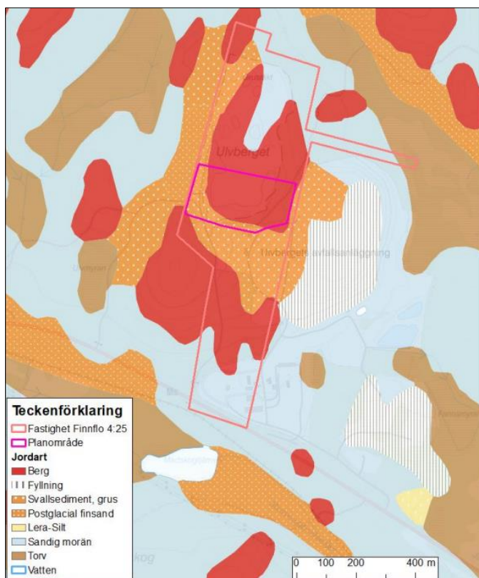
Figur 11, Jordarter inom planområdet, berg (röd), morän (blå) och postglacial sand (orange med större prickar).
