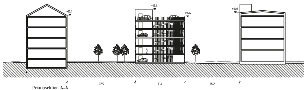
Bild 19. Sektion Drottninggatan- Östra Hamngatan.
