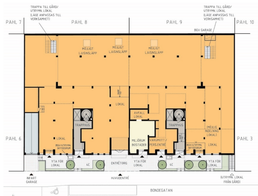
Förslag på entréplan med utrymme för 600 kvadratmeter tillkommande bruttoarea (BTA) för lokaler (Total arkitektur).
