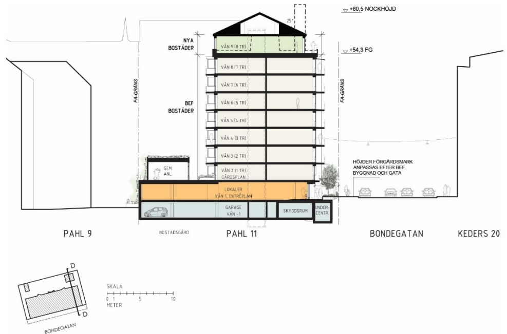
Sektion som illustrerar utrymmet mellan Pahl 9 och Pahl 11 (Total arkitektur).
