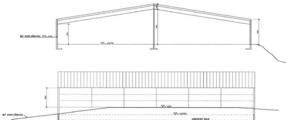
Sektion och fasad: nedsänkt tennisanläggning på växthusplatsen
