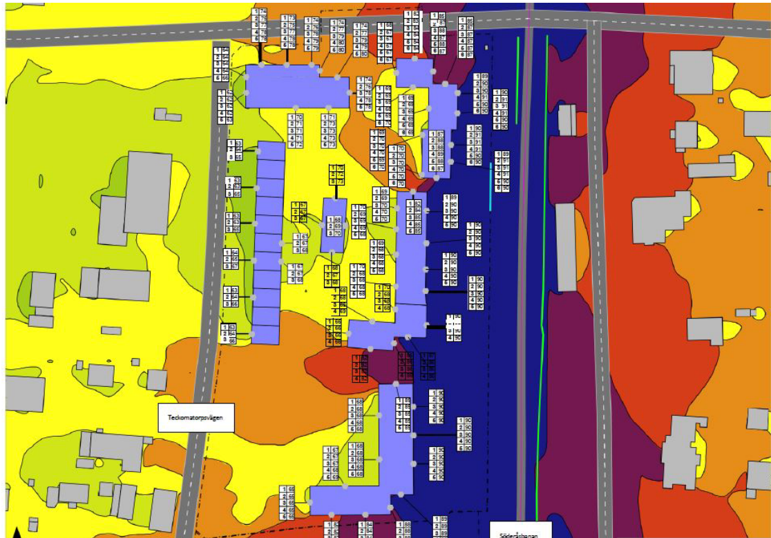
Bild ovan visar resultat från beräkning av maximala ljudnivåer vid godstågspassage. Ljundnivå 2 meter övermark samt frifältsvärden vid fasad. Förekommer år 2040 ca 14 ggr per dygn, vara 3-4 ggr under nattetid, med 20 meter lång bullerskärm.
