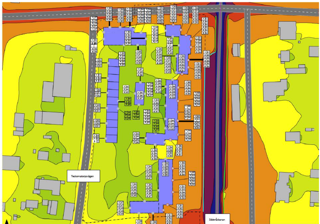
Bild ovan visar resultat från beräkning av sammanvägd ljudnivå från tåg- och vägtrafik som bygger på prognos för år 2040, med en 2,5 meter hög bullerskärm vid planområdesgräns till järnvägen. Ljundnivå 2 meter övermark samt frifältsvärden vid fasad. Ekvivalenta ljudnivåer.
