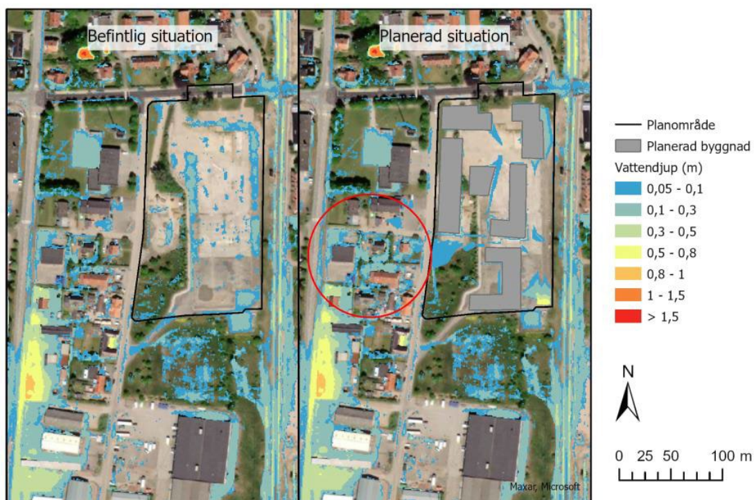
Bilden visar skillnaden mellan befintlig och planerad situation vid ett 100-års regn.
