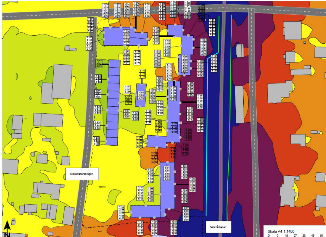
Bild ovan visar resultat från beräkning av maximala ljudnivåer vid godstågspassage som bygger på prognos för år 2040, med en 2,5 meter hög bullerskärm vid planområdesgräns till järnvägen. Ljudnivå 2 meter över mark samt frifältsvärden vid fasad. Ekvivalenta ljudnivåer.
