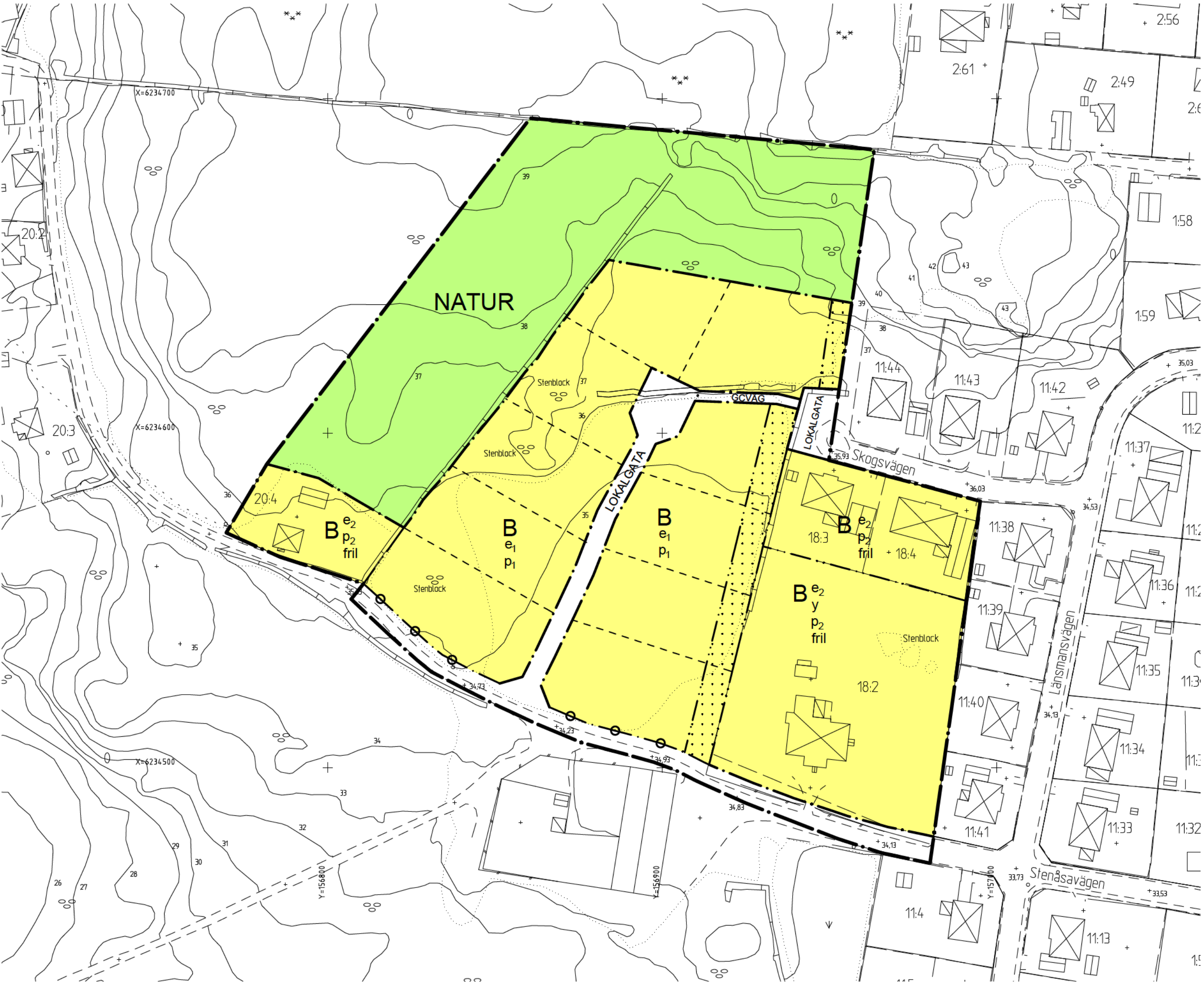
PLANKARTA 1:1000
