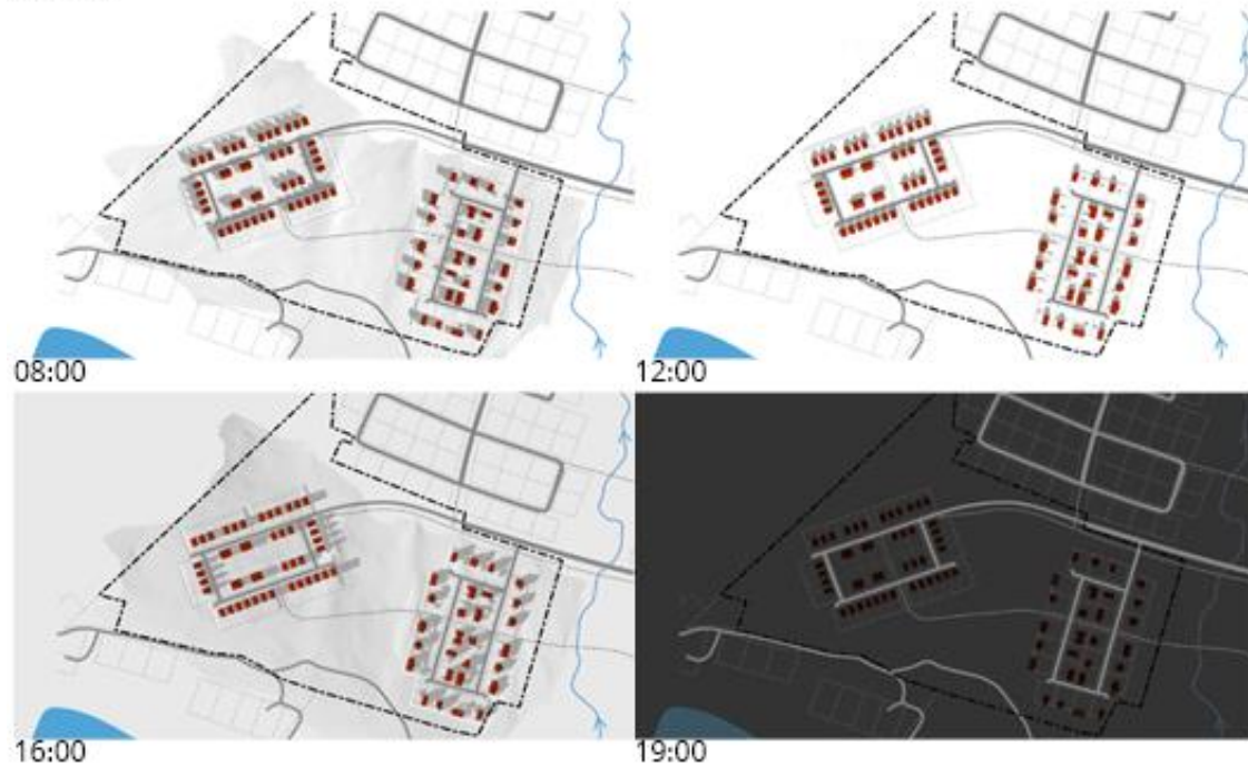
Figur 10. Skuggeffekter 1 april.
