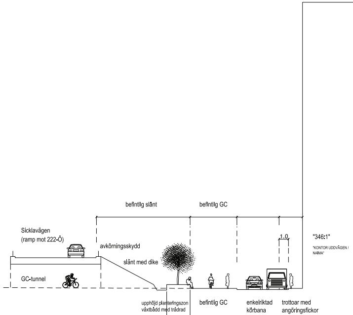
GATUSEKTION D-D 1:400
