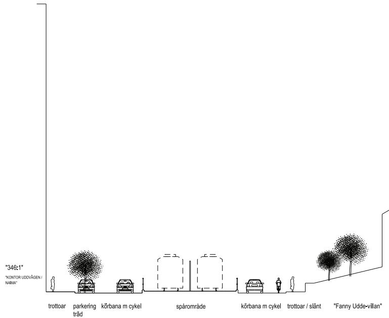
GATUSEKTION G-G 1:400
