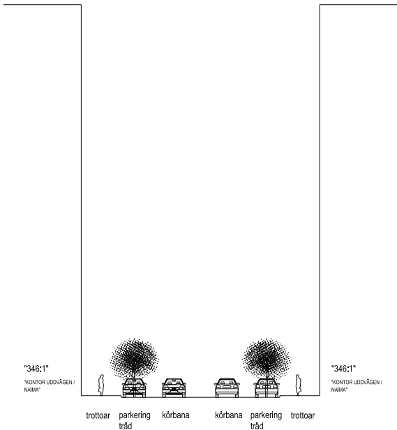
GATUSEKTION C-C 1:400
