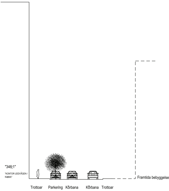
GATUSEKTION E-E 1:400
