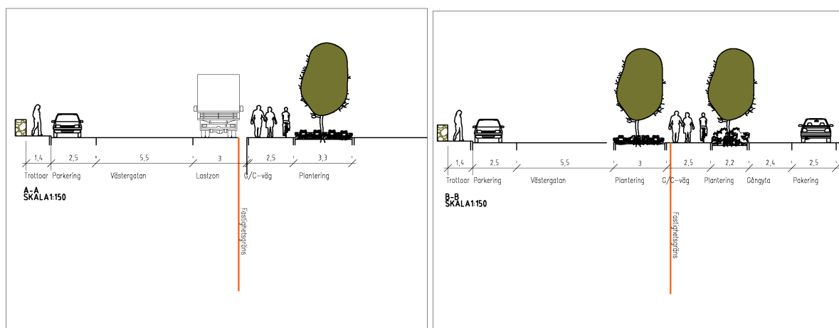
Figur 2. Sektion A-A och B-B över Västergatan visar hur gång- och cykelbanan kommer innanför dagens fastighetsgräns.
