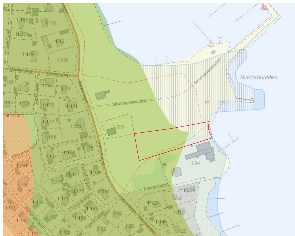
Kartutdrag som visar jordarter SGU, med planområde markerat i rött.
