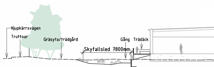
Figur 35. Illustration som visar en sektion av föreslagen flödesväg för skyfallsvatten i form av ett dike väster om skolbyggnaden. Sektionen är markerad i illustrationsplanen ovan som A-a (Novaterra).
