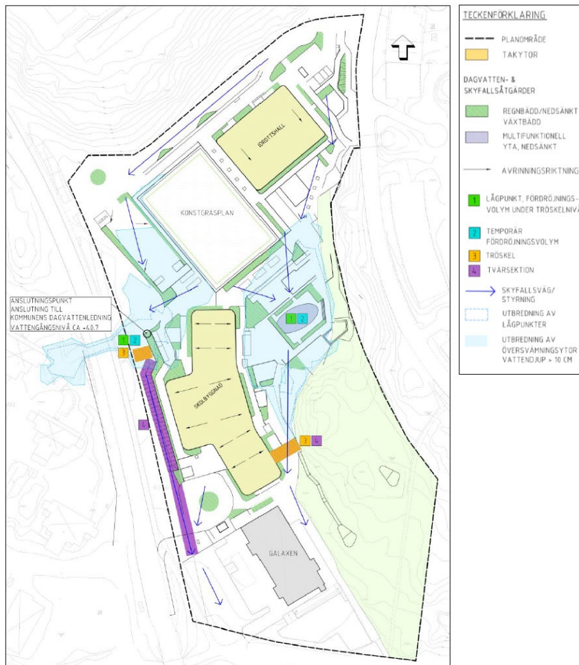
Figur 32. Avvattningsplan som visar principlösning för skyfall- och dagvattenhantering. (Sweco).
