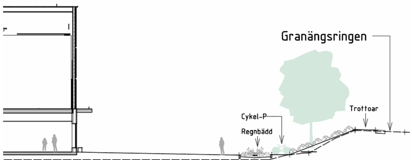
Figur 14. Föreslagen sektion som visar nivåskillnaden mellan platsen öster om idrottsbollen och Granängsringen (Novaterra).
