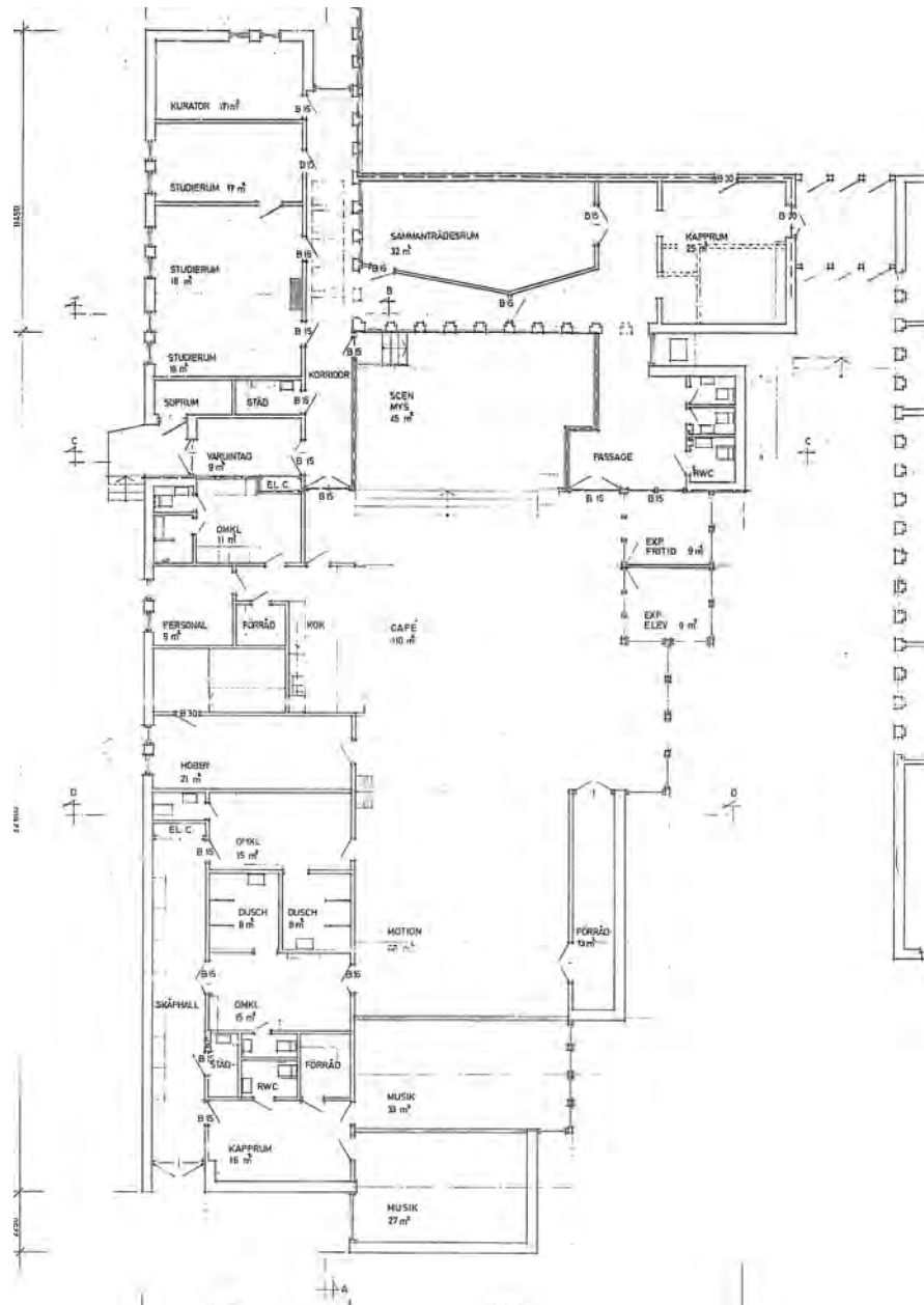
Högstadieskola, tillbyggnad fritidsgård, plan BV, arkitekt K-Konsult 1978
