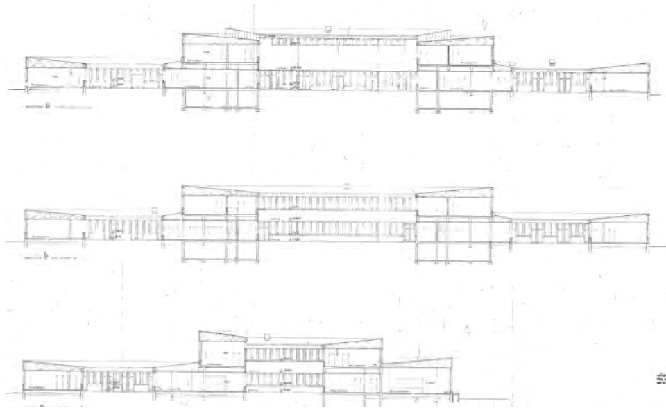
Högstadieskola, huvudbyggnad, sektioner
