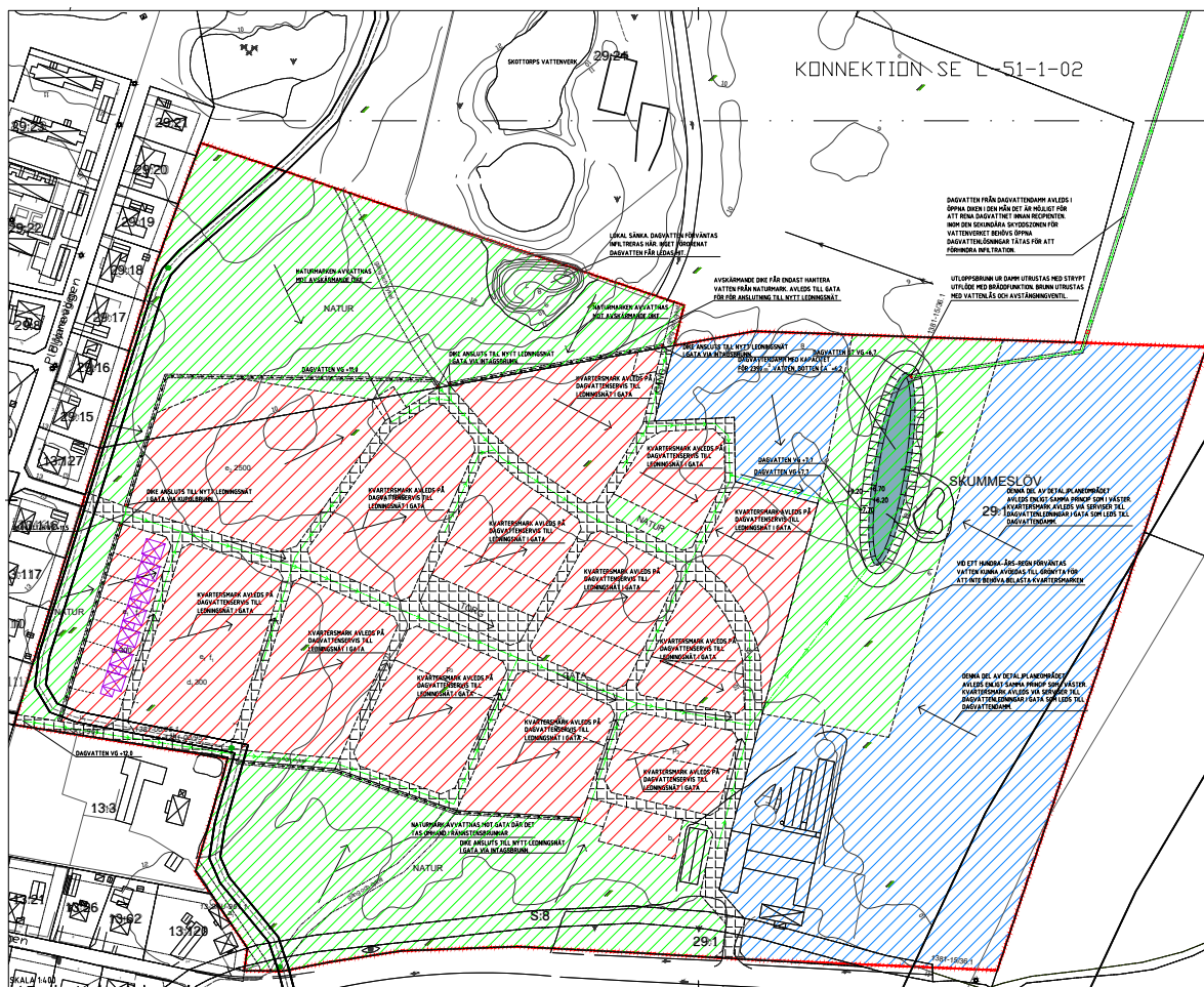
Figur 29: Föreslagna dagvattenlösningar.
