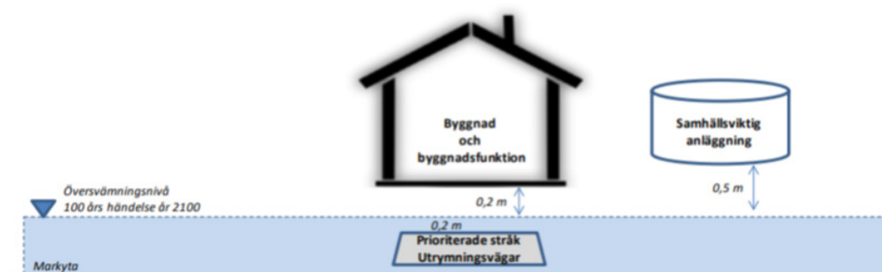
Figur 3. Exempel på visualisering av planeringsnivåer vid skyfall (Göteborgs Stad, Stadsbyggnadskontoret 2019).
