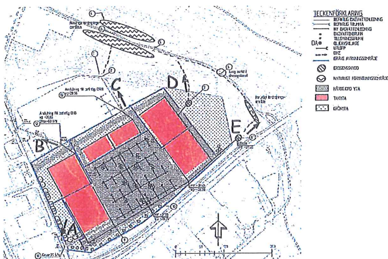
Föreslaget avrinningsområde för Veddesta 2:83, den mellersta bygganden har utgått i föreskriven plan. Tyréns
